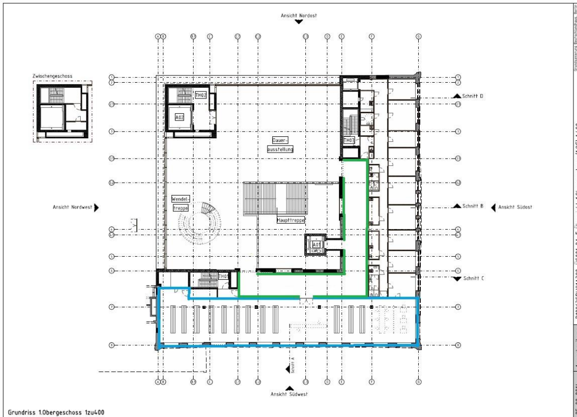
Abb. 1: Grundriss erstes Obergeschoss mit Bibliothek & Zeitzeugenarchiv (blau) und Wandelgang (grün)
